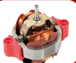
Motore PRO AC fabbricato in Italia
